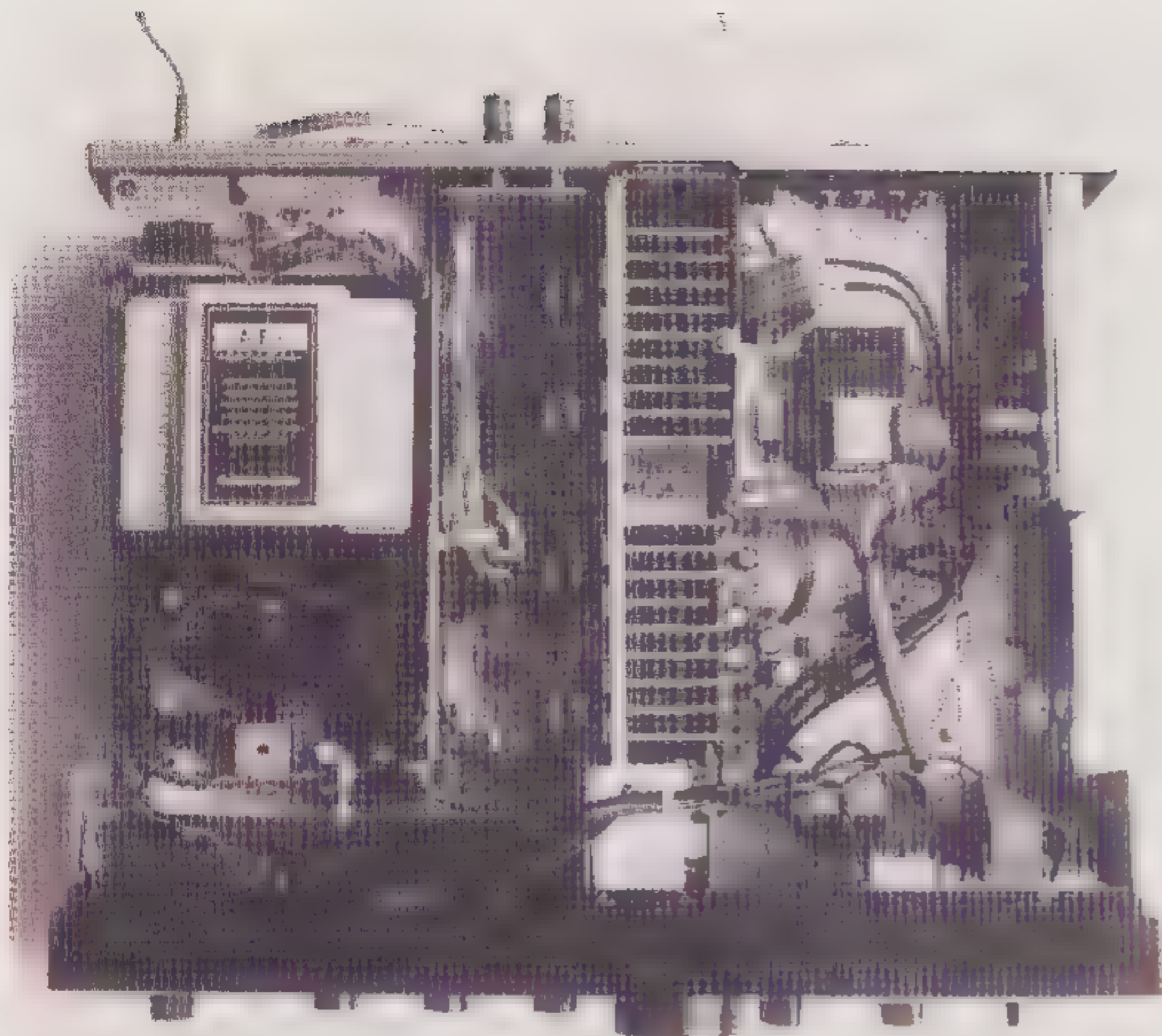
Op de foto zien we links de zeer forse AEI voedingstransformator. Midden rechts is de via een motortje gestuurde ALPS keuzeschakelaar te zien.
